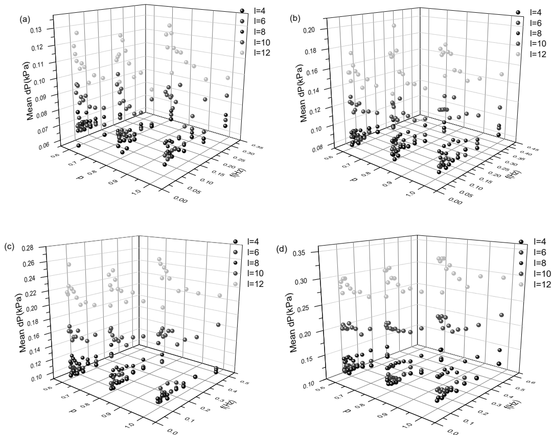
(a) Q=80\text{ml/s} , Re=300 ; (b) Q=100\text{ml/s} , Re=375 ; (c) Q=120\text{ml/s} , Re=425 ; (d) Q=140\text{ml/s} , Re=525
