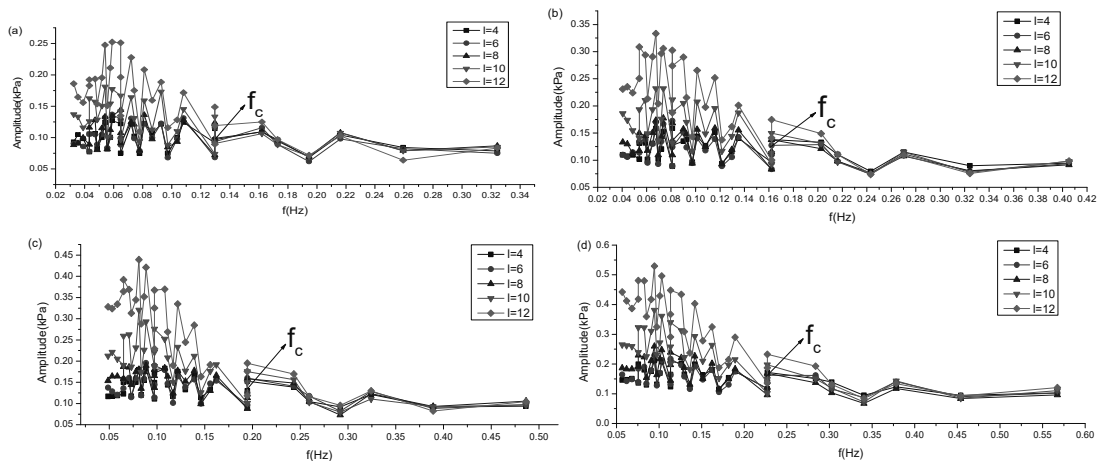
(a) Q_s=80\text{ml/s} , Re=300 ; (b) Q_s=100\text{ml/s} , Re=375 ; (c) Q_s=120\text{ml/s} , Re=450 ; (d) Q_s=140\text{ml/s} , Re=525
